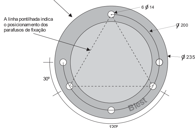
BASE - PLANTA
