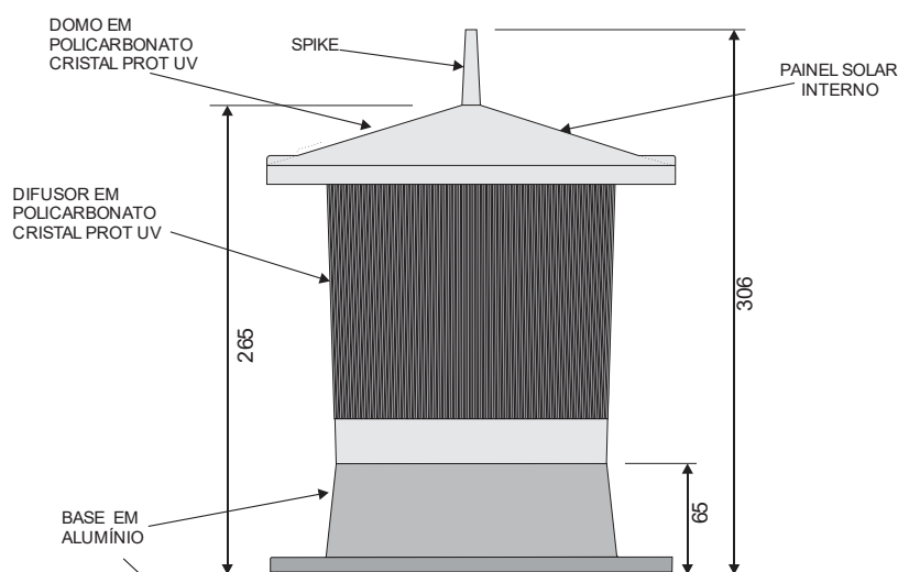
LANTERNA - PERFIL
